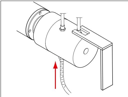
Abb. 8: Anschluss der Leckageleitung planen
